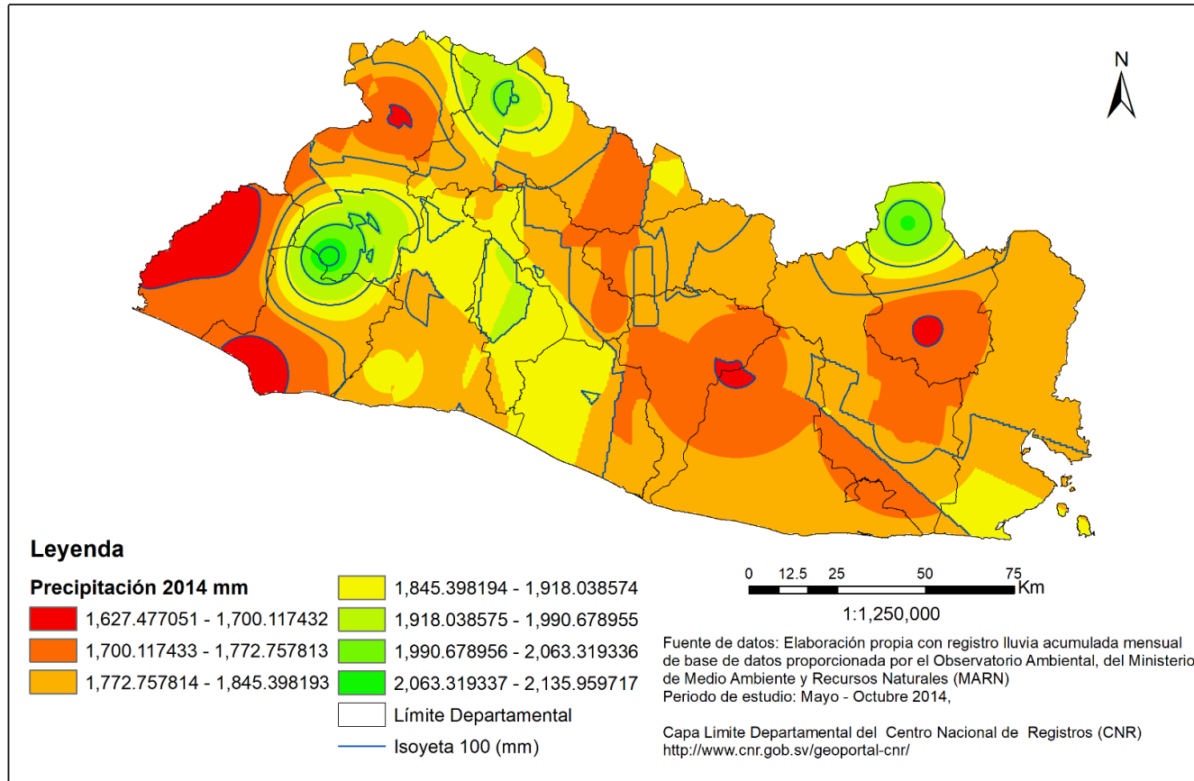
Figura 40. Mapa de precipitación, año 2014 Fuente: Elaboración propia.
