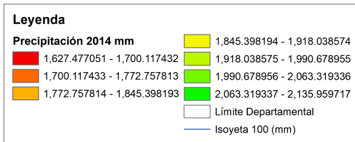
Figura 52. Mapa de precipitación, zona oriental, año 2014. Fuente: Elaboración propia.
