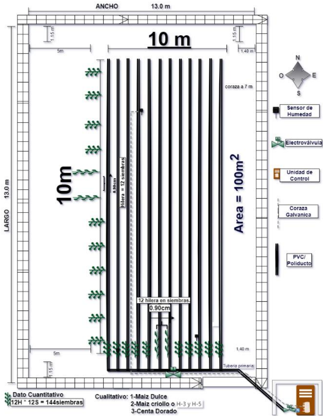
Figura 13. Diagrama integrado del prototipo del sistema riego Chalatenango.
