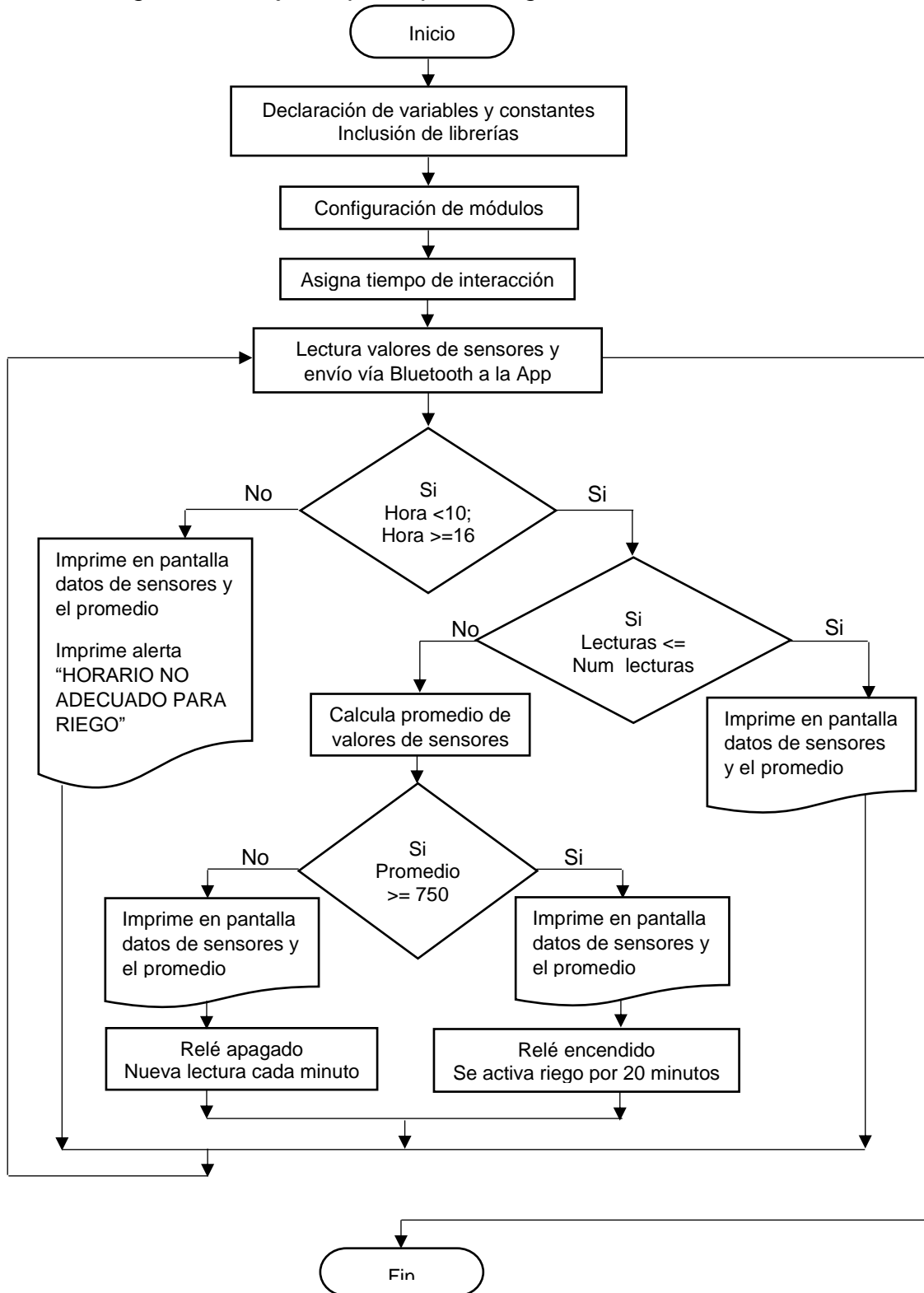
Figura 15. Diagrama de flujo del prototipo de riego.
