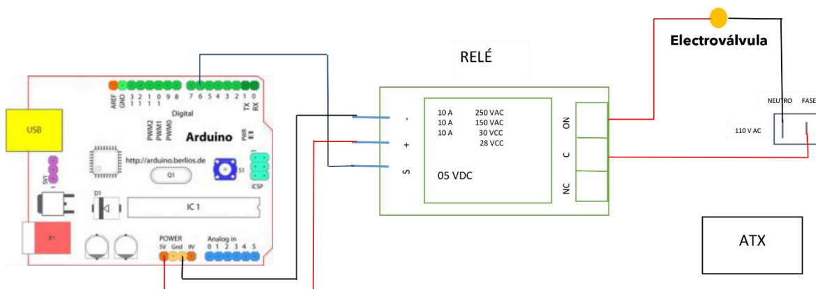
Figura 11. Diagrama de conexión de electroválvula con relé y la placa Arduino.
