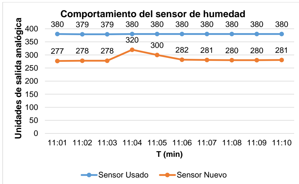
Figura 19. Resultados de prueba de dos sensores de humedad de suelo en tierra húmeda.
