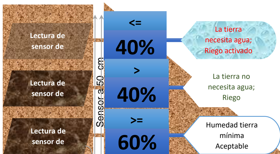
Figura 23. Porcentaje de humedad del suelo para activación de riego.
