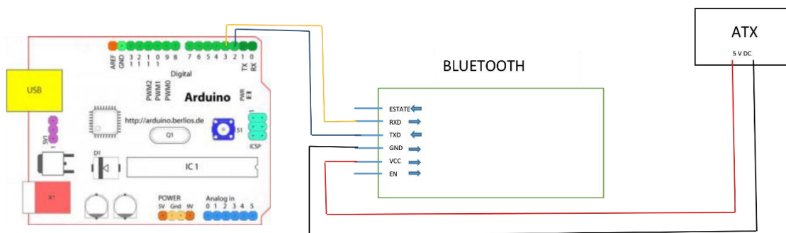
Figura 12. Conexión y adaptación de la electroválvula con relé y la placa Arduino.
