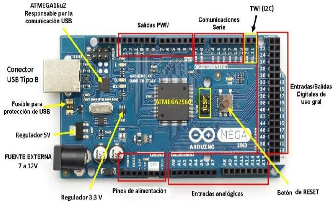
Figura 2. Modelo de placa Arduino Mega 2560
