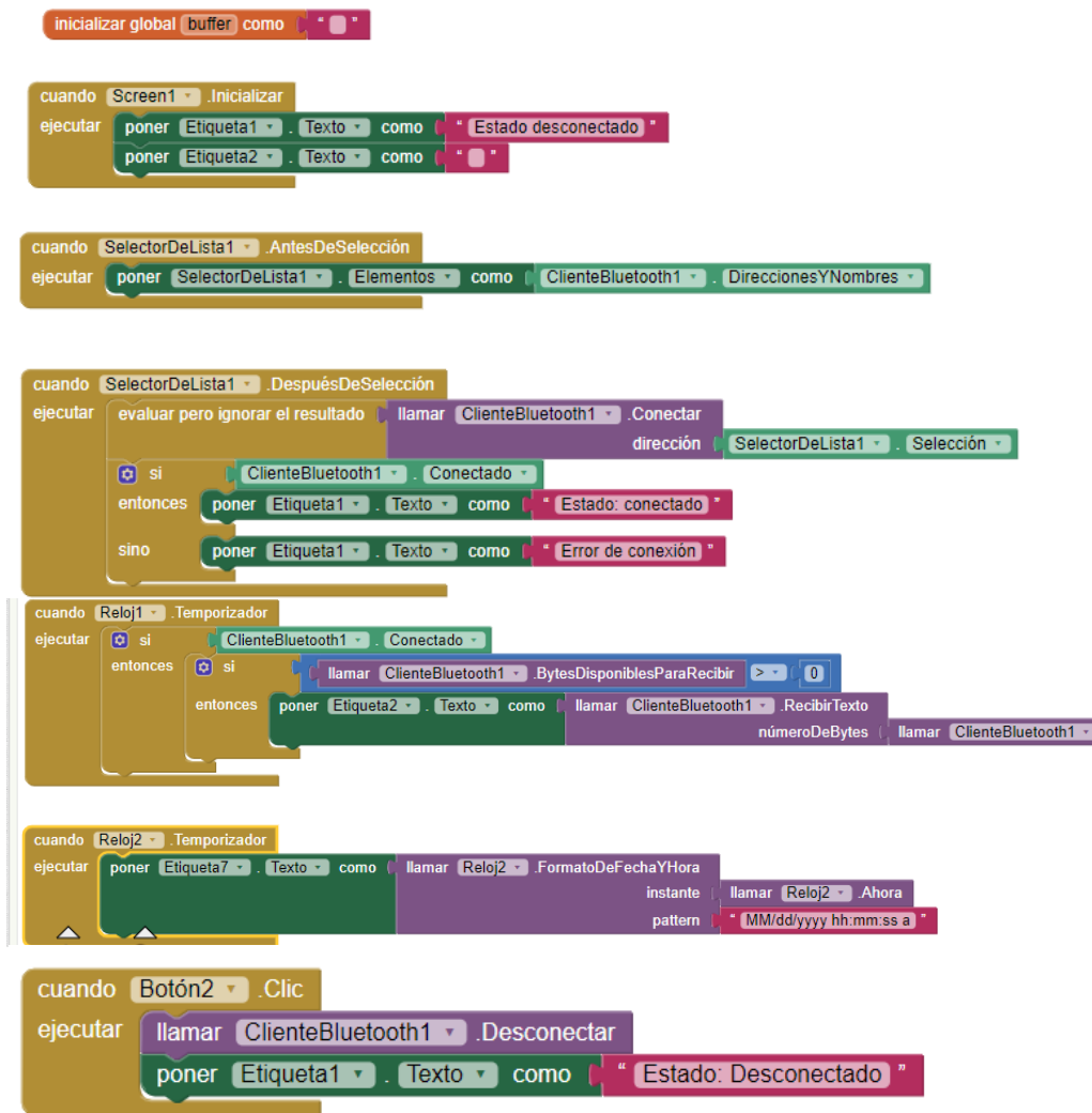
Figura 30. Codificación de aplicación móvil.
