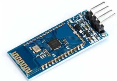
Figura 9. Modulo Bluetooth.
