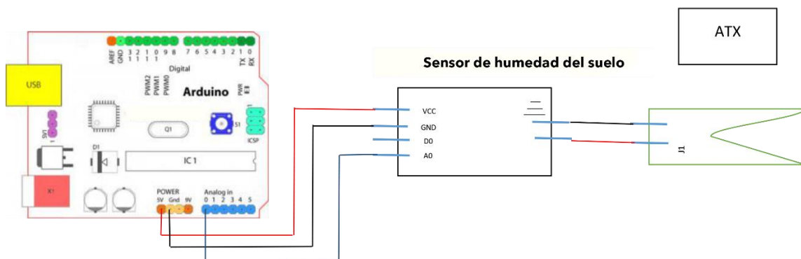
Figura 10. Diagrama de conexión de sensores.
