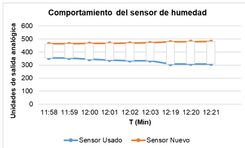
Figura 21. Resultado de prueba de dos sensores de humedad de suelo en tierra subhúmeda.
