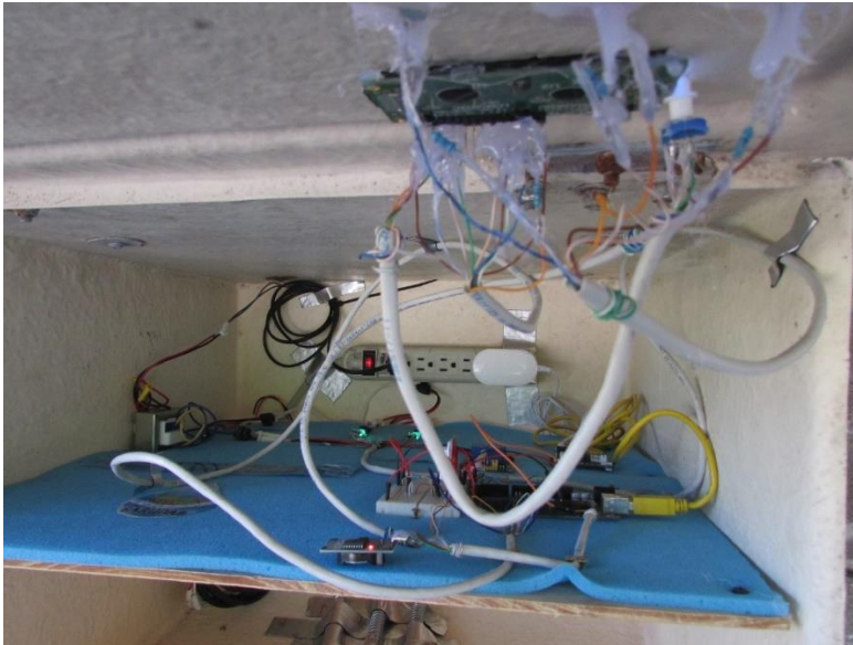
Figura 27. Instalación de unidad de control en parcela de Chalatenango.
