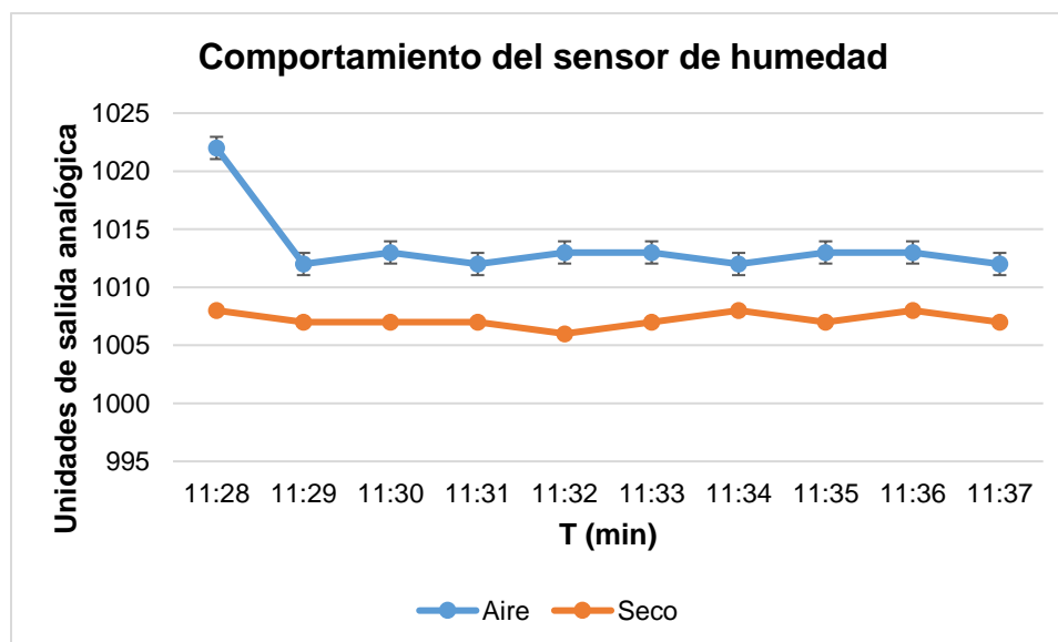
Figura 17. Resultados de prueba de sensor de humedad de suelo en diferente ambiente.
