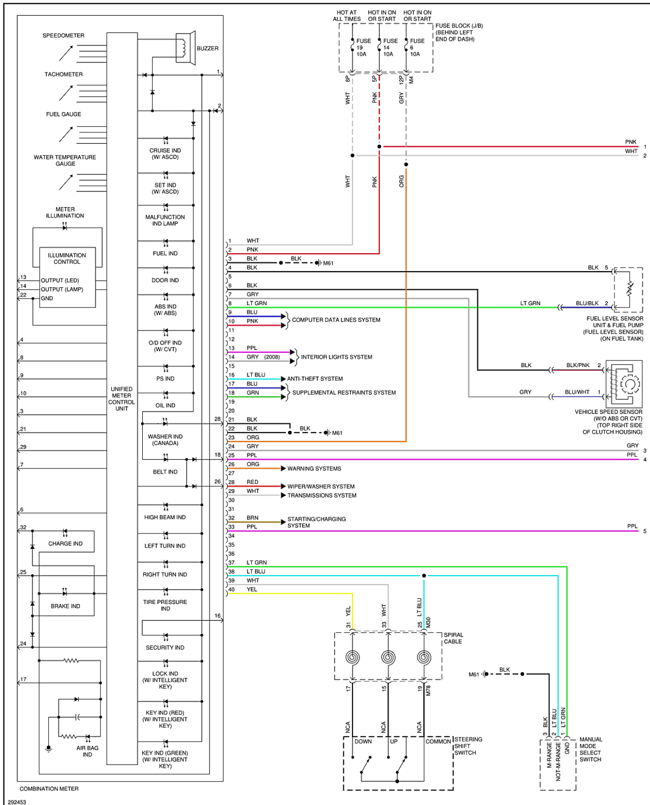
Fig. 41. Esquema de conexión de panel de instrumentos - Parte 1.
