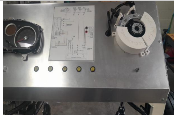
Vista preliminar de componentes panel frontal.
