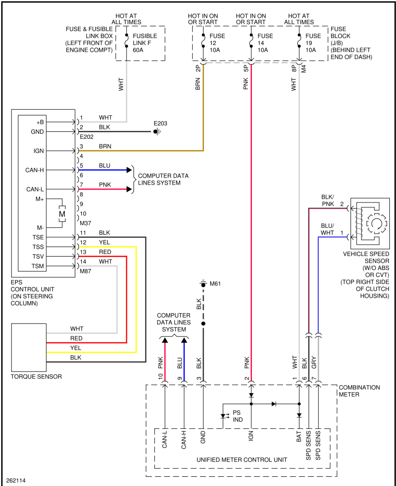
Fig. 29. Esquema de control de sistema de dirección asistida eléctricamente.
