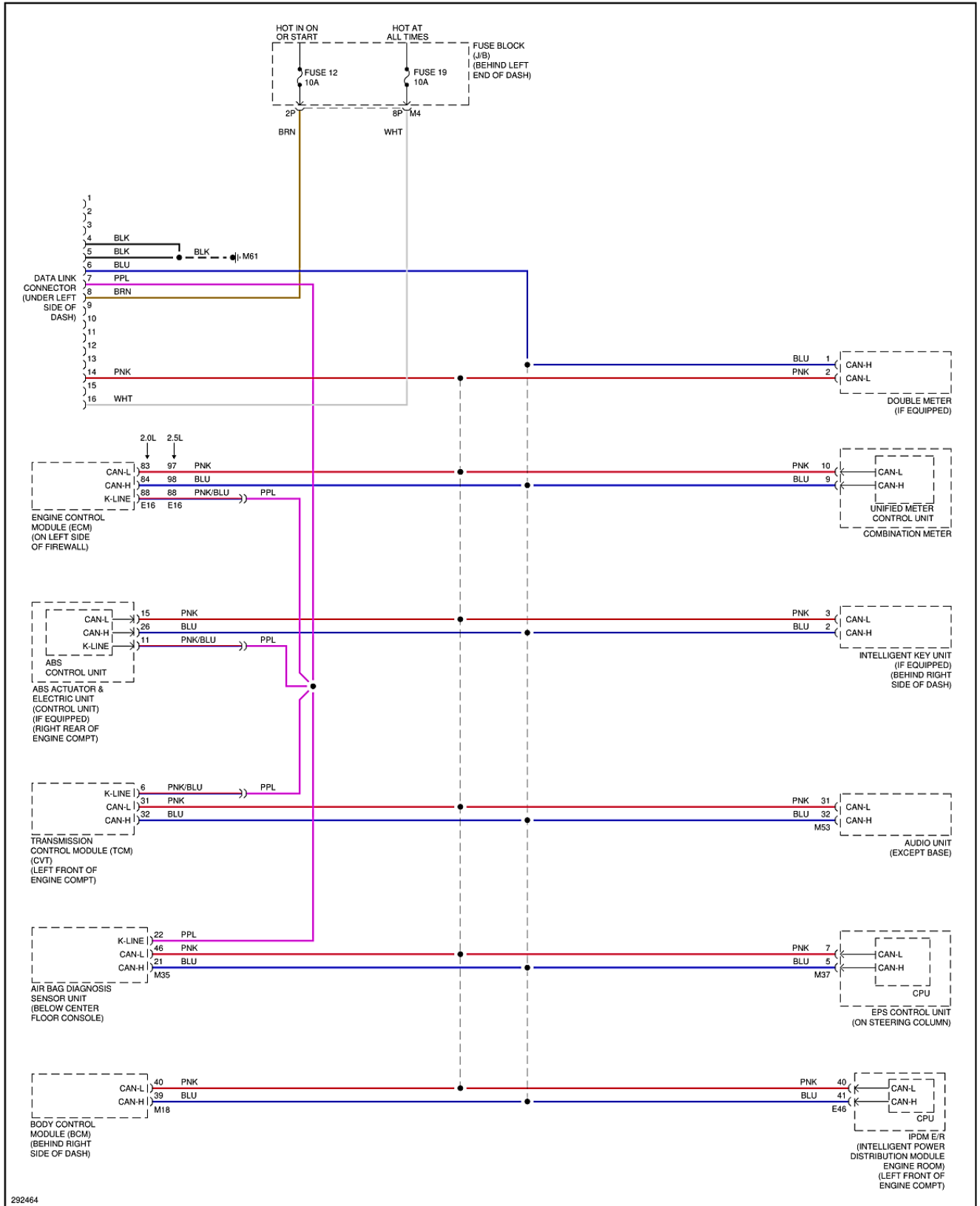
Fig. 32. Esquema de conexión de módulos de control red CAN-bus.
