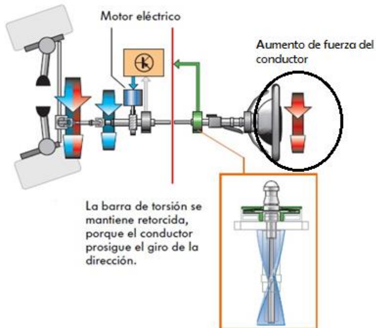
Fig. 25. Aumento de fuerza y asistencia eléctrica.
