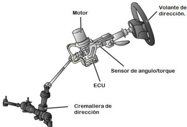
Fig. 11. Ubicación de componentes eléctricos y mecánicos.
