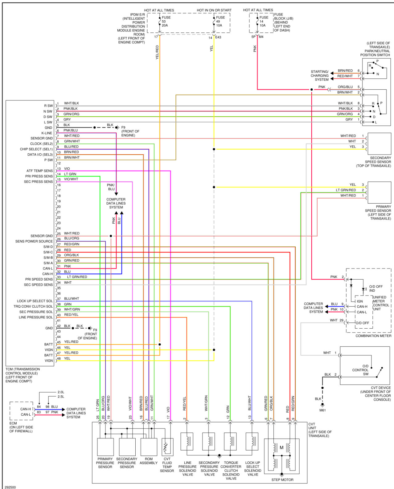
Fig. 45. Esquema de conexión de módulo de control de transmisión TCM.
