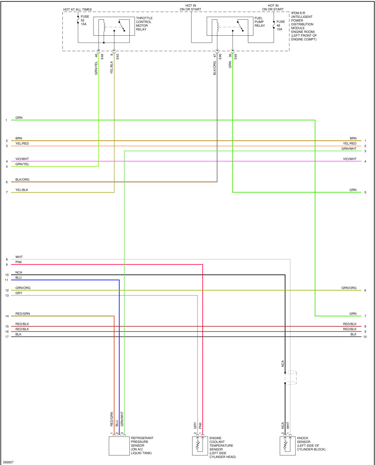
Fig. 35. Esquema de conexión de los elementos en el sistema de motor Nissan Sentra 2008 - Parte 3.
