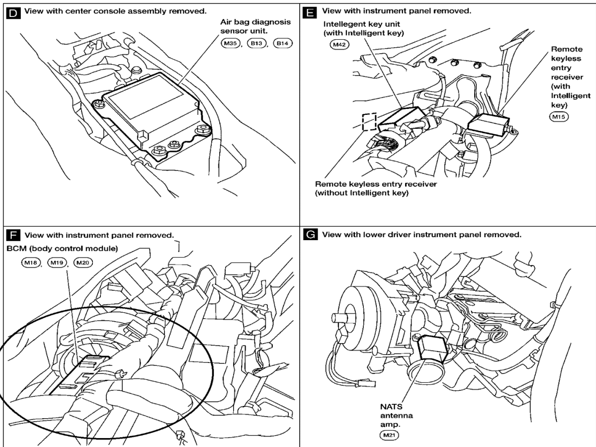
Fig. 40. Identificación de BCM y ubicación del componente.
