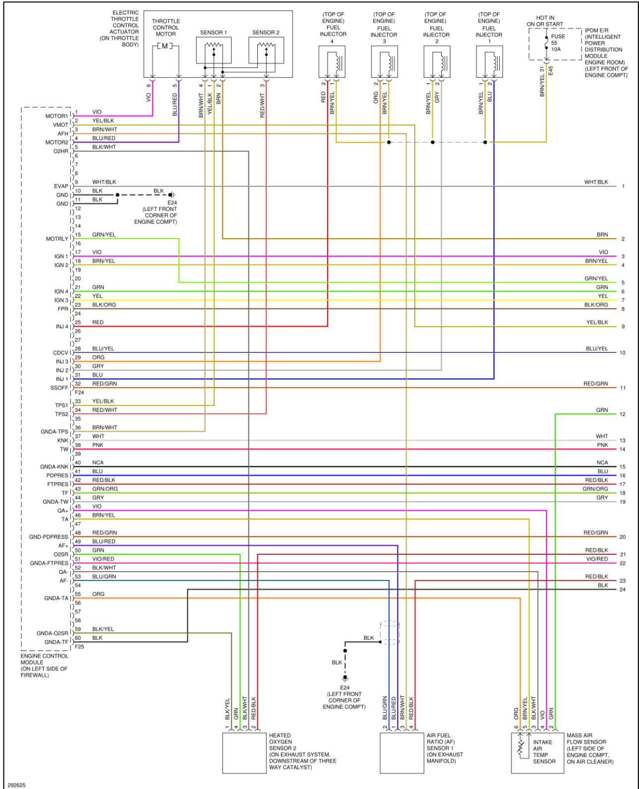
Fig. 33. Esquema de conexión de los elementos en el sistema de motor Nissan Sentra 2008 - Parte 1.
