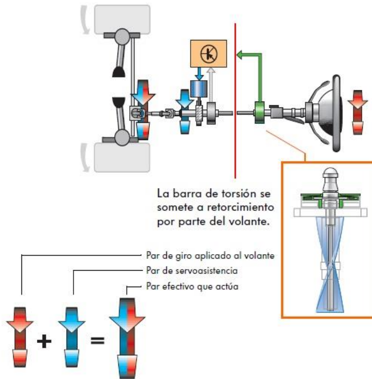
Fig. 24. Esquema de funcionamiento con asistencia eléctrica.
