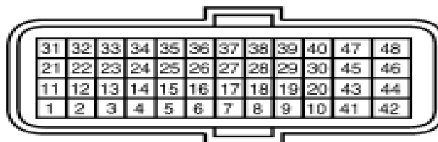
Fig. 46. Ubicación e identificación de pines de módulo de control de transmisión TCM.
