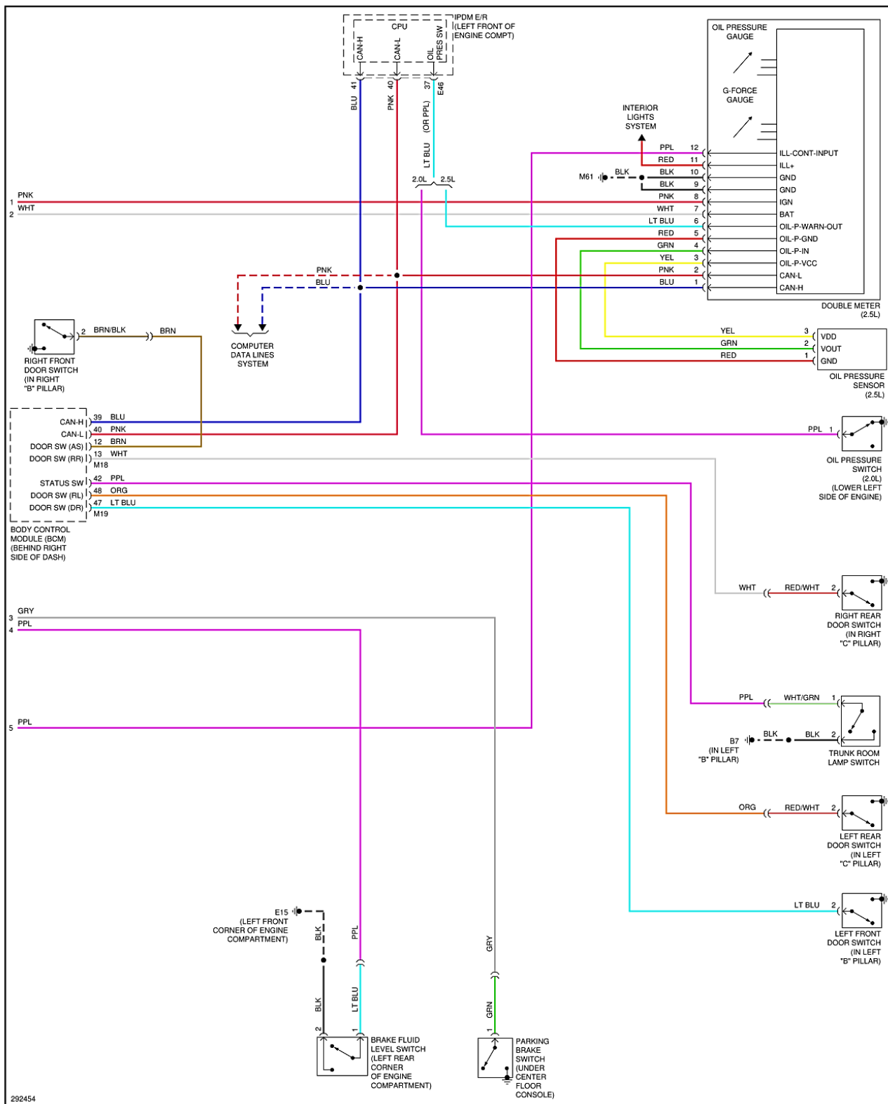
Fig. 42. Esquema de conexión de panel de instrumentos - Parte 2.
