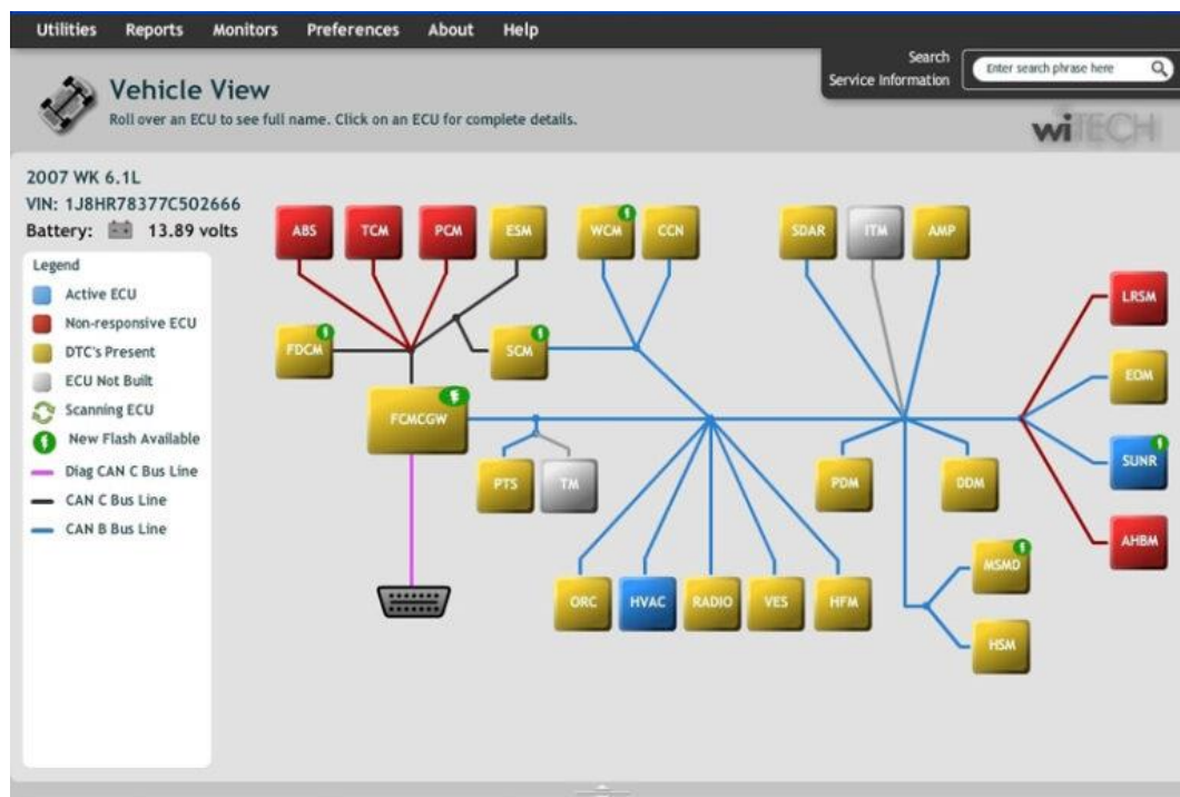
Fig. 6. Ejemplo de mapa topológico de red electrónica de comunicación.
