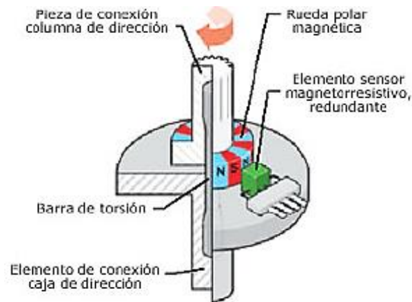
Fig. 20. Esquema de un sensor de par.
