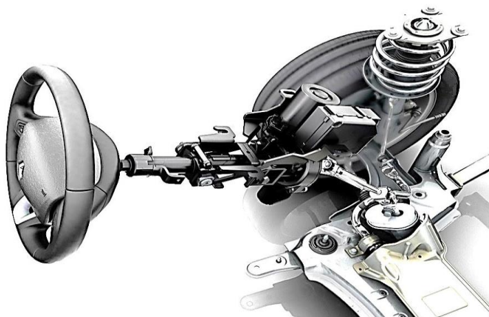
Fig. 8. montaje de un sistema de dirección asistida eléctricamente. EPS.
