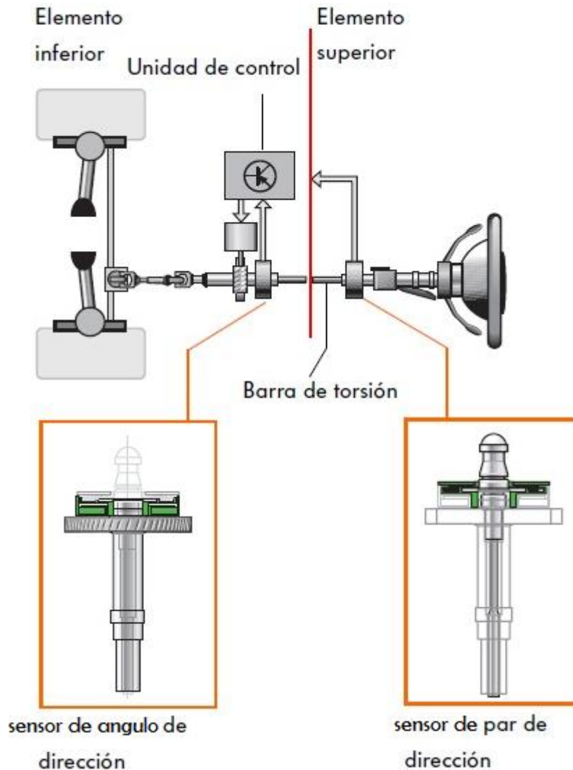
Fig. 23. Esquema de funcionamiento de elementos mecánicos y eléctricos.
