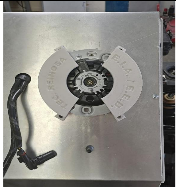
Impresión 3D de protectores de reluctor.
