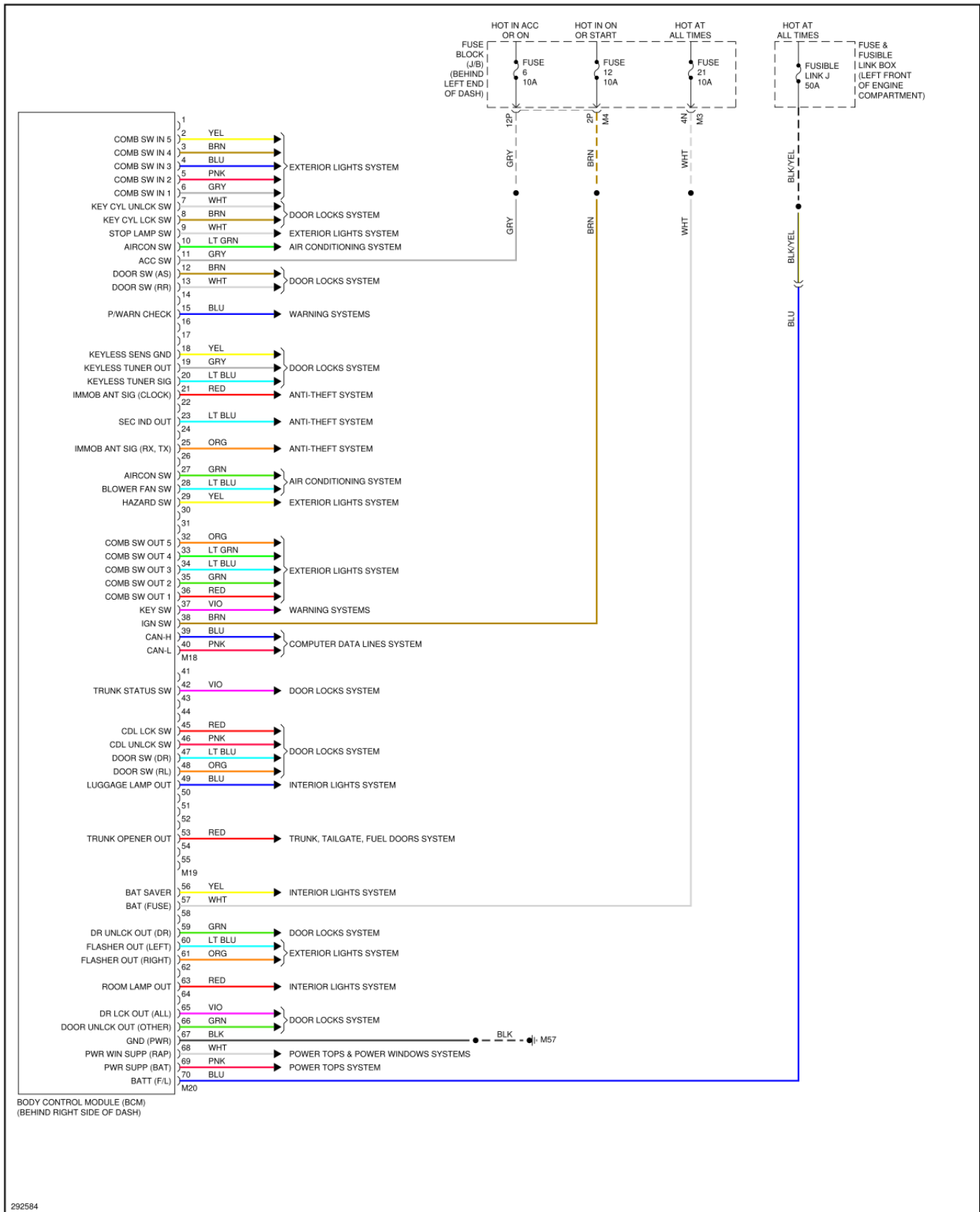
Fig. 39. Esquema eléctrico de módulo de control de carrocería
