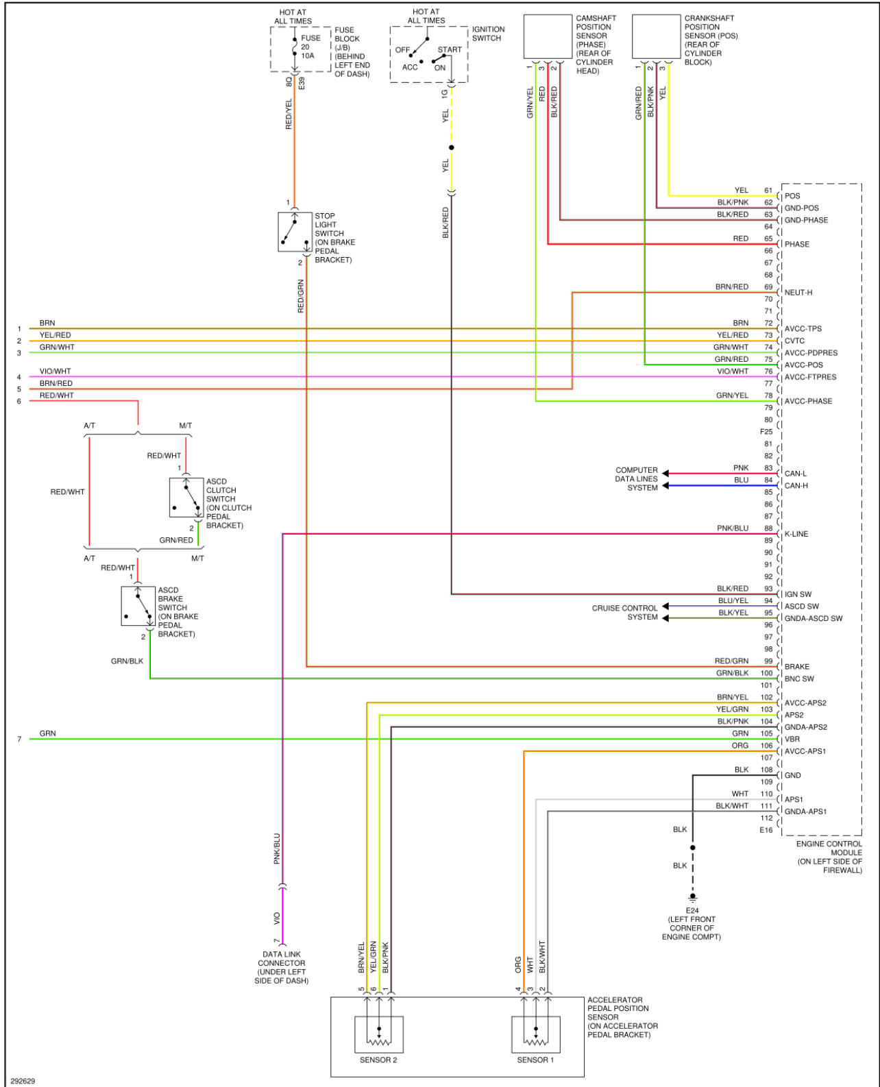
Fig. 37. Esquema de conexión de los elementos en el sistema de motor Nissan Sentra 2008 - Parte 5.
