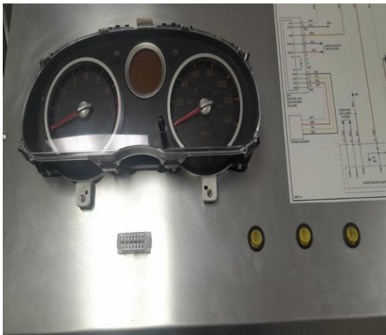
Instalación de conector de diagnostico e interruptores de simulacion de fallas.
