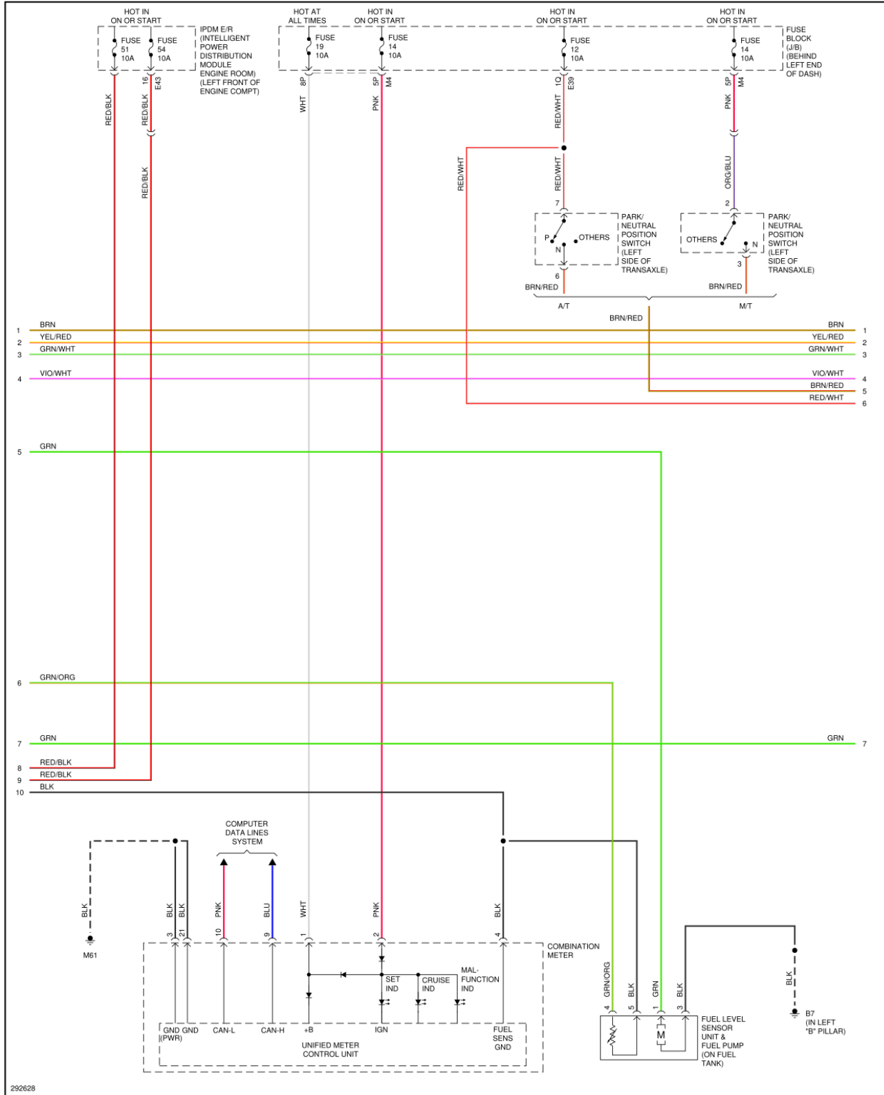
Fig. 36. Esquema de conexión de los elementos en el sistema de motor Nissan Sentra 2008 - Parte 4.
