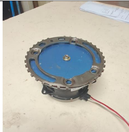
Montaje preliminar de reluctor en motor.
