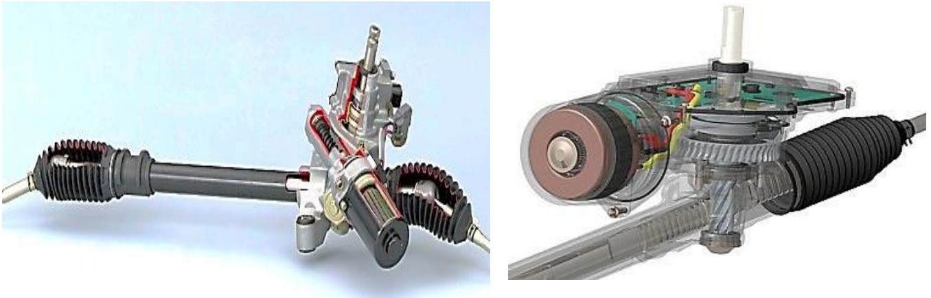
Fig. 14. Montaje de motor eléctrico entre la columna de dirección y la cremallera.
