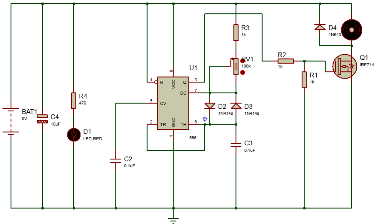
Fig. 28. Esquema de control de variador de velocidad motor DC.
