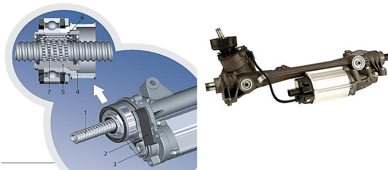
Fig. 15. Montaje de motor eléctrico en la cremallera de dirección.
