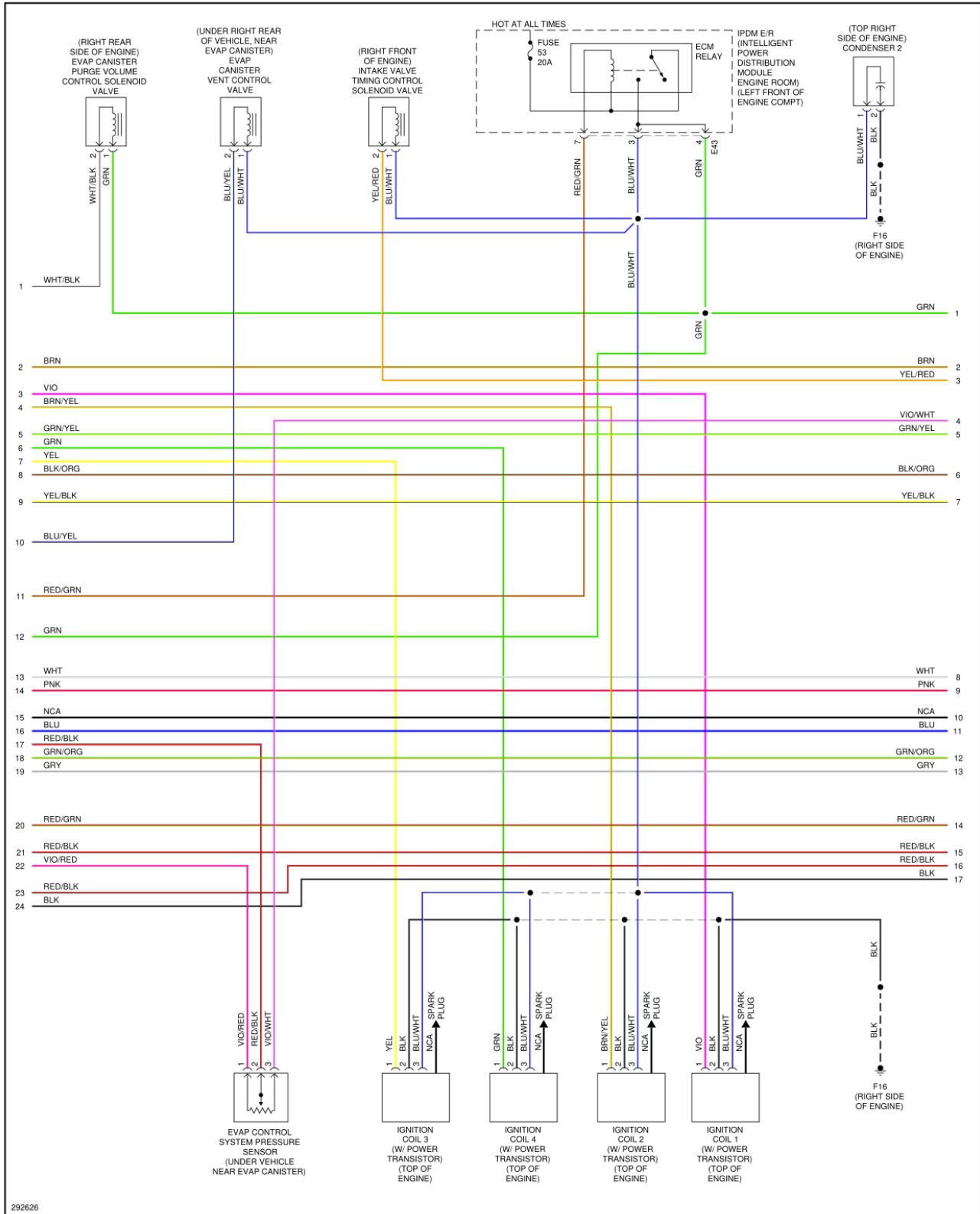
Fig. 34. Esquema de conexión de los elementos en el sistema de motor Nissan Sentra 2008 - Parte 2.
