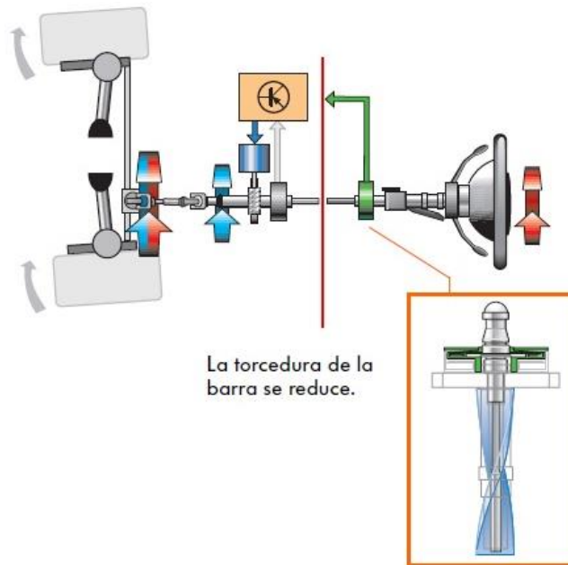
Fig. 26. Reducción de fuerza en el volante.
