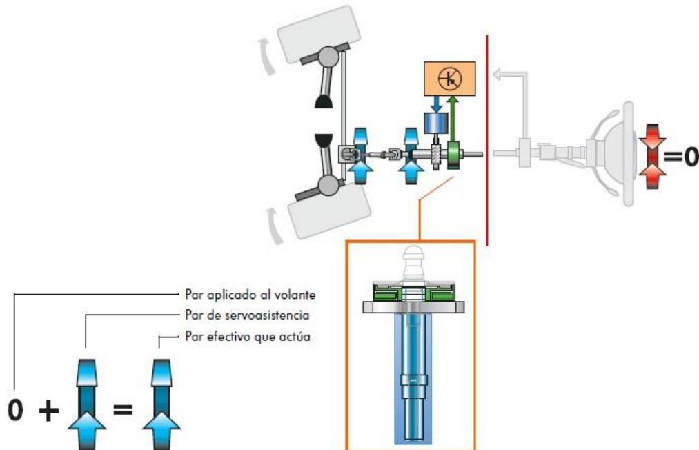
Fig. 27. Función de retro giro activo.
